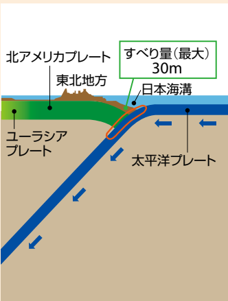
震源過程解析から推定された、断面上のすべり量分布
