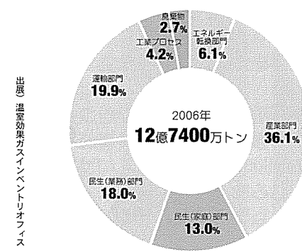
(グラフ2) 日本の部門別二酸化炭素排出量 ～各部門の割合～
