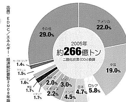
(グラフ1) 世界の二酸化炭素排出量 ～国別排出割合～
