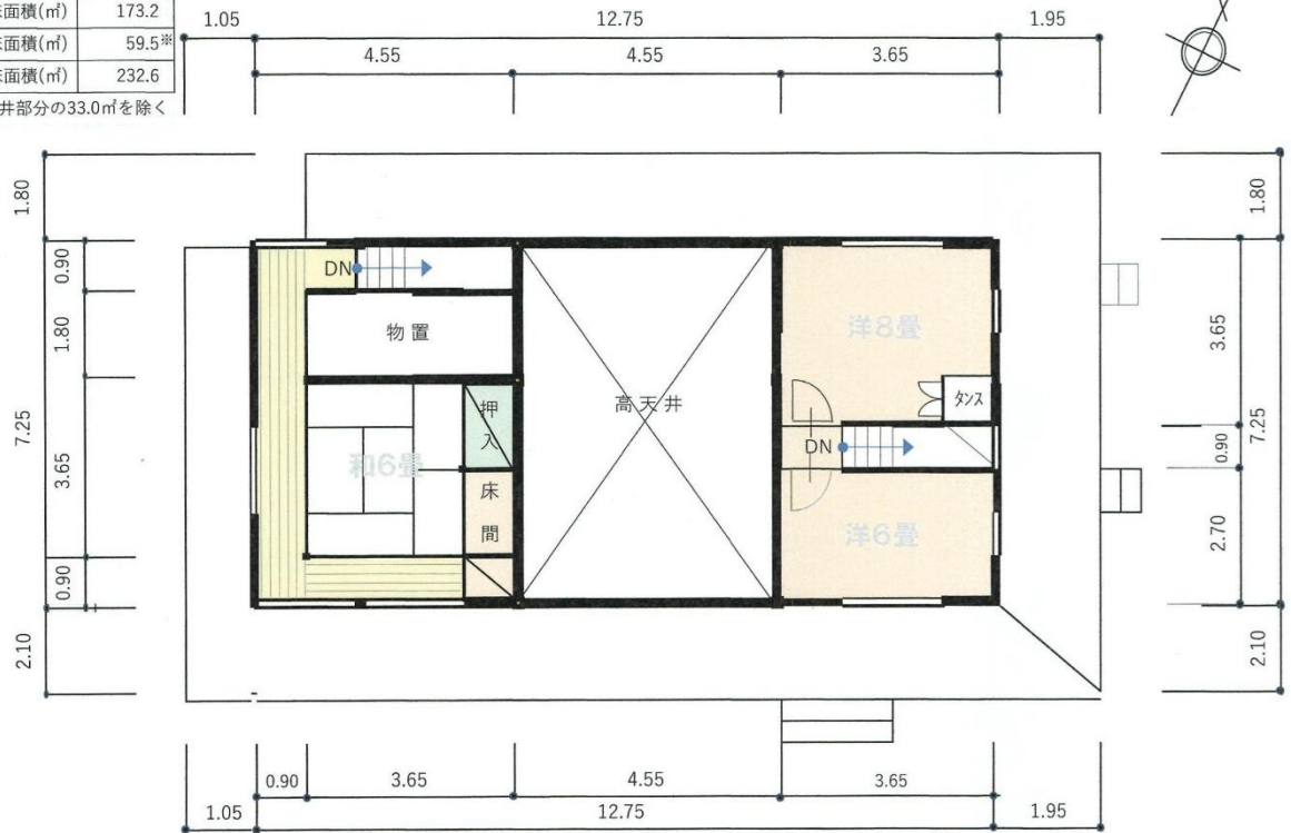
2階間取図
