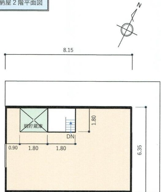
納屋 2階平面図
