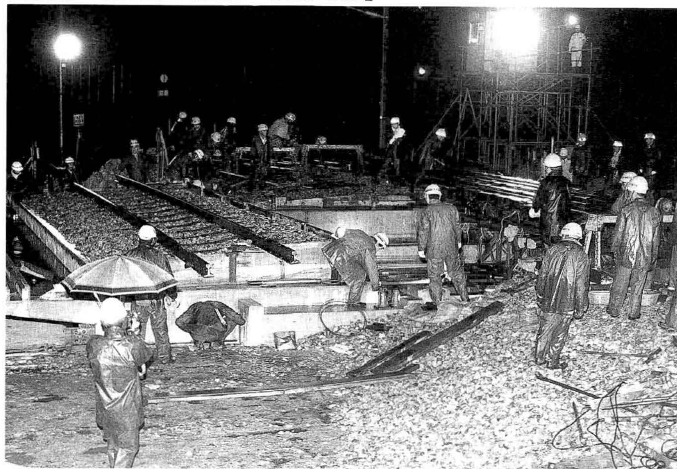
▲泊桜町線とJR立体交差部の桁付け換え工事(6月21日午前2時～)
