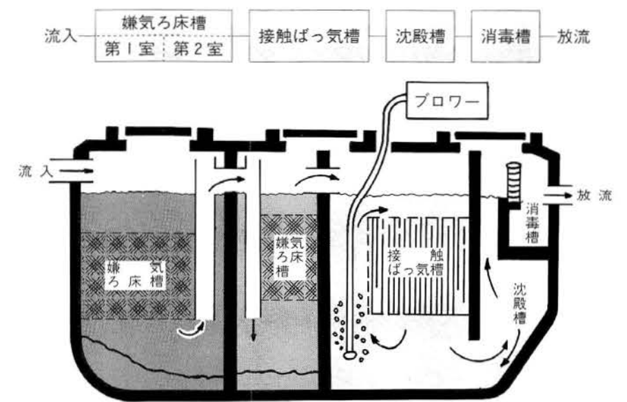
■図3 合併処理浄化槽のしくみ
