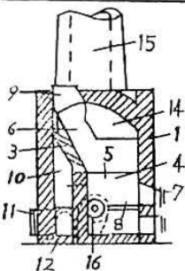
横断側面図
